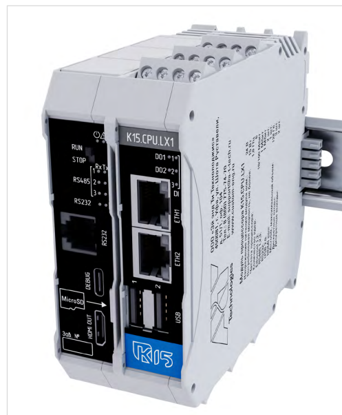
Внешний вид контроллера «K15.CPU.LX1»
