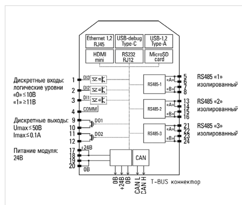
Схема подключения
