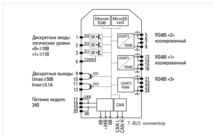
Схема подключения
