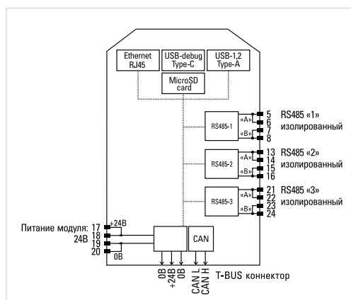
Схема подключения
