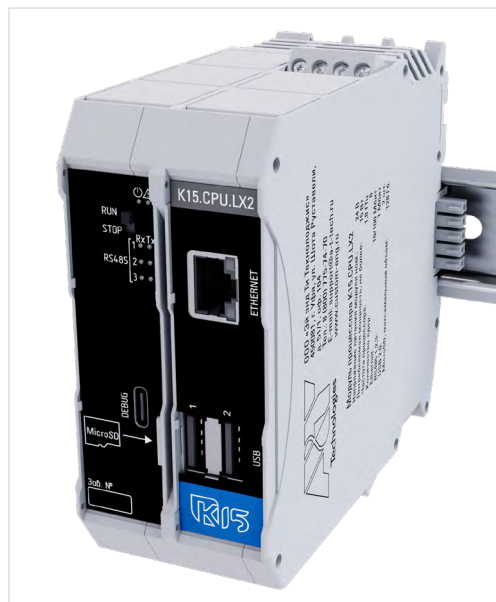
Внешний вид контроллера «K15.CPU.LX2»
