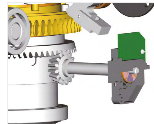
ДАТЧИК ПОЛОЖЕНИЯ
